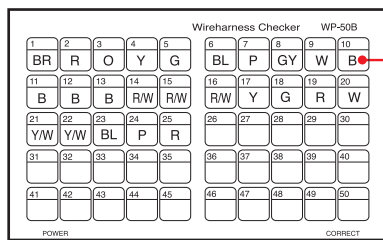
線色・回路番号を記入
